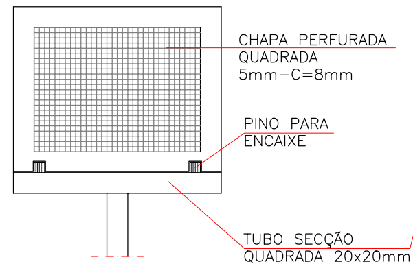
CORTE ESCALA 1:5
