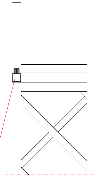
DETALHE ESCALA 1:5
