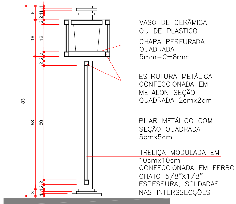
CORTE ESCALA 1:10
