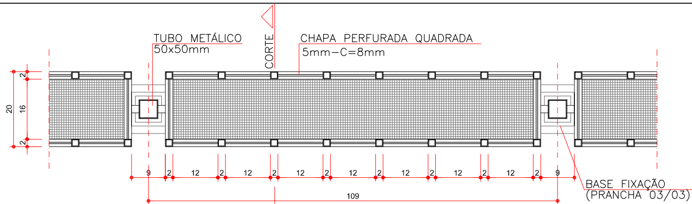
PLANTA ESCALA 1:10
