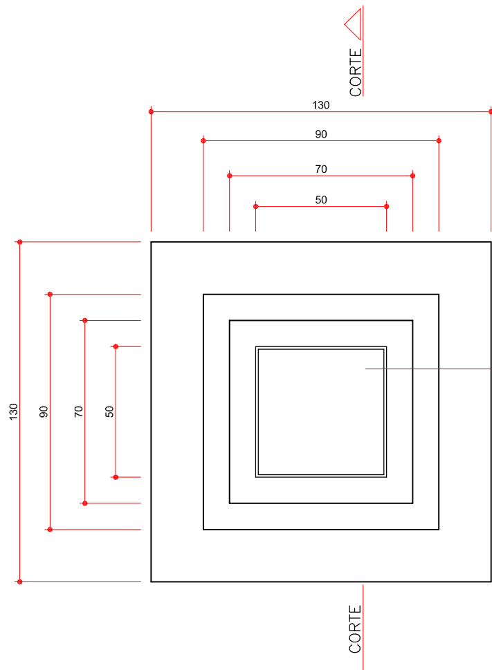
BASE DE FIXAÇÃO PLANTA ESCALA 1:2
