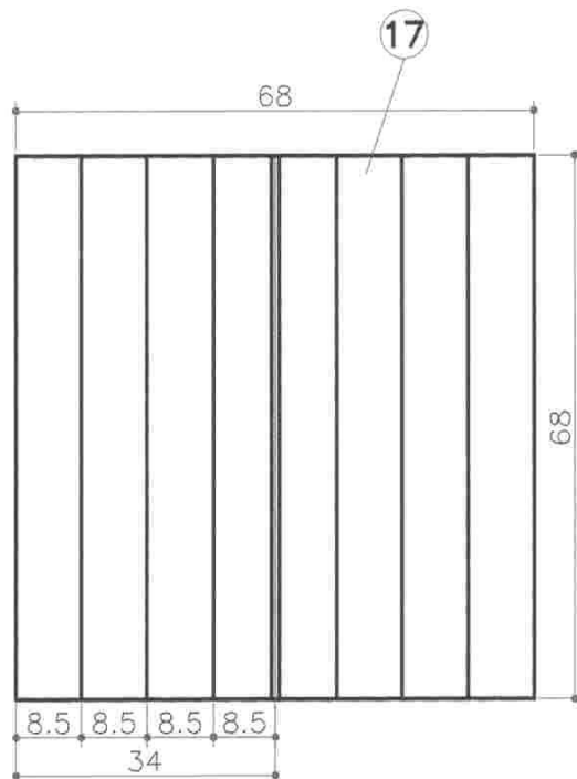
VISTA SUPERIOR
