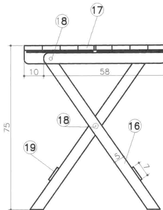
VISTA LATERAL
