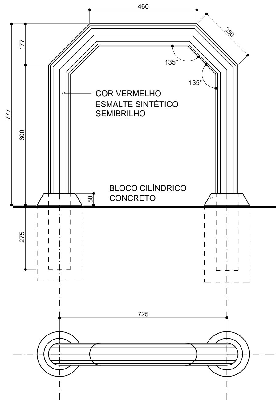
PLANTA CORRIMÃO TUBO MECÂNICO STANDARD (INDUSTRIAL). DIÂMETRO 3 1/2" - MSG - 16 - 1,5mm.
