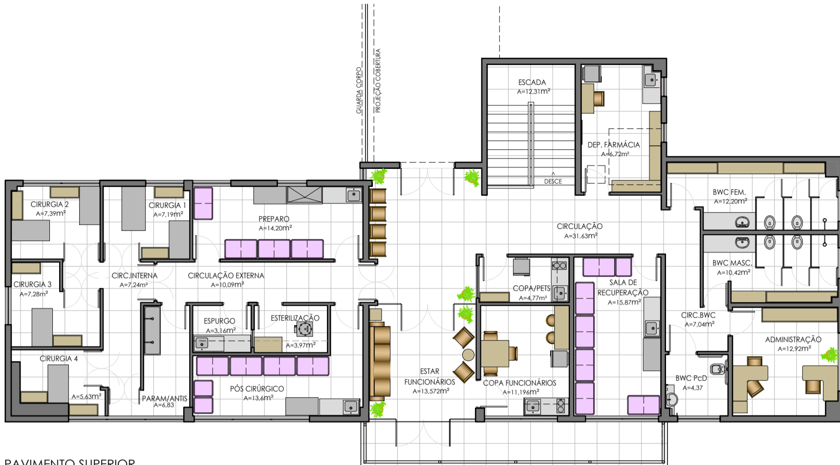
PAVIMENTO SUPERIOR ÁREA 256,62m 2 ESCALA: 1/125
